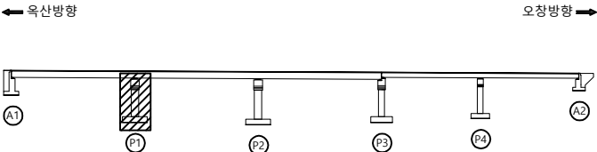
배면
